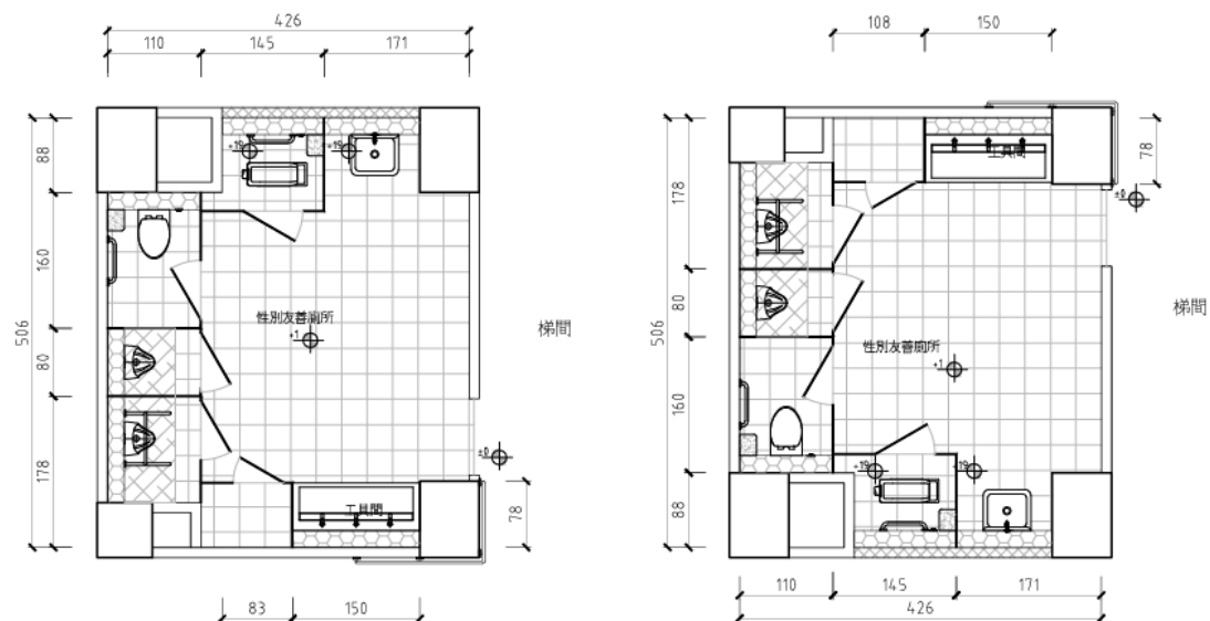
性別友善廁所平面圖 A3-S-1/54 單位：CM
